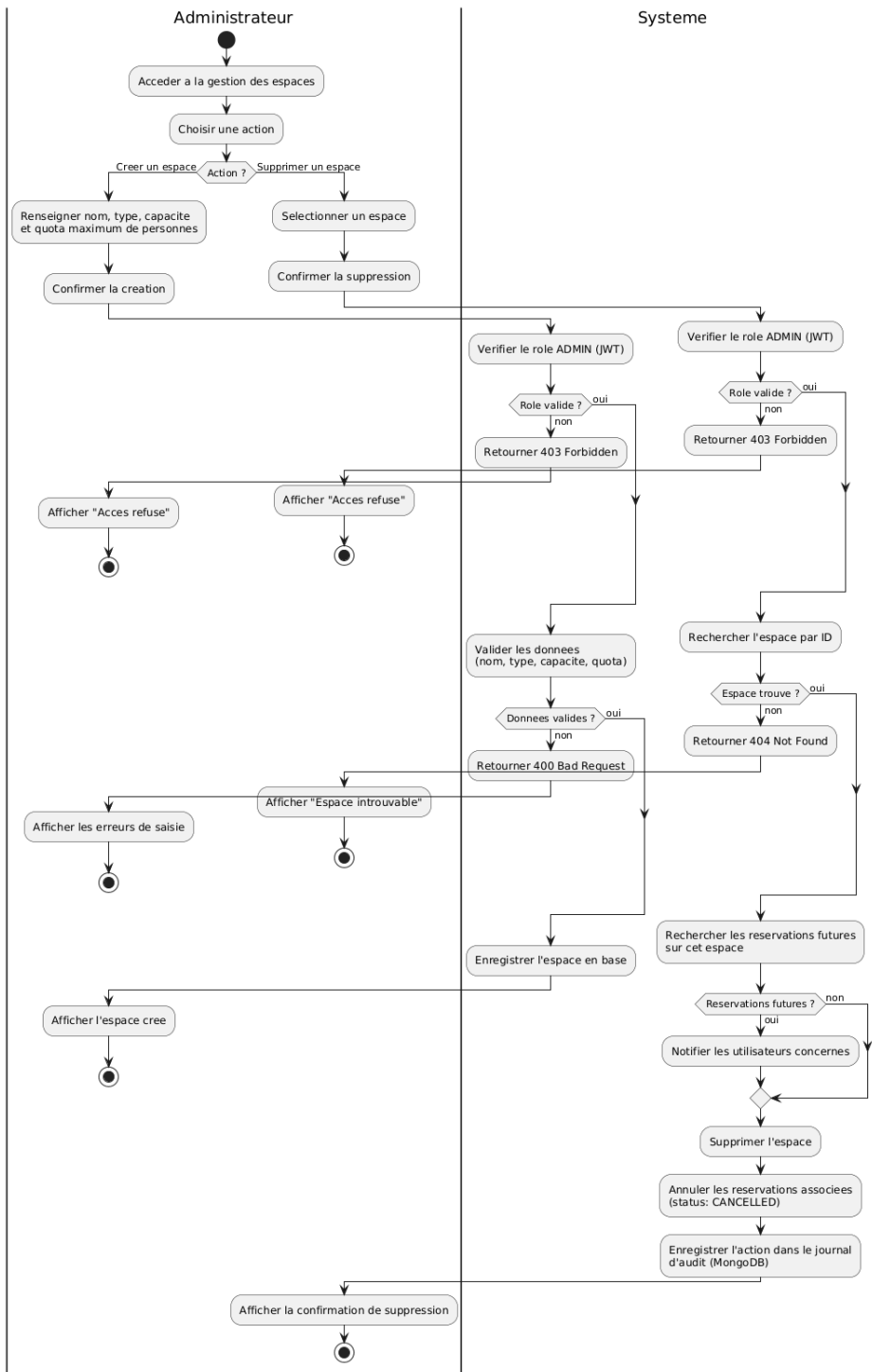
Diagramme d'activité - Gestion des espaces (Administrateur)
